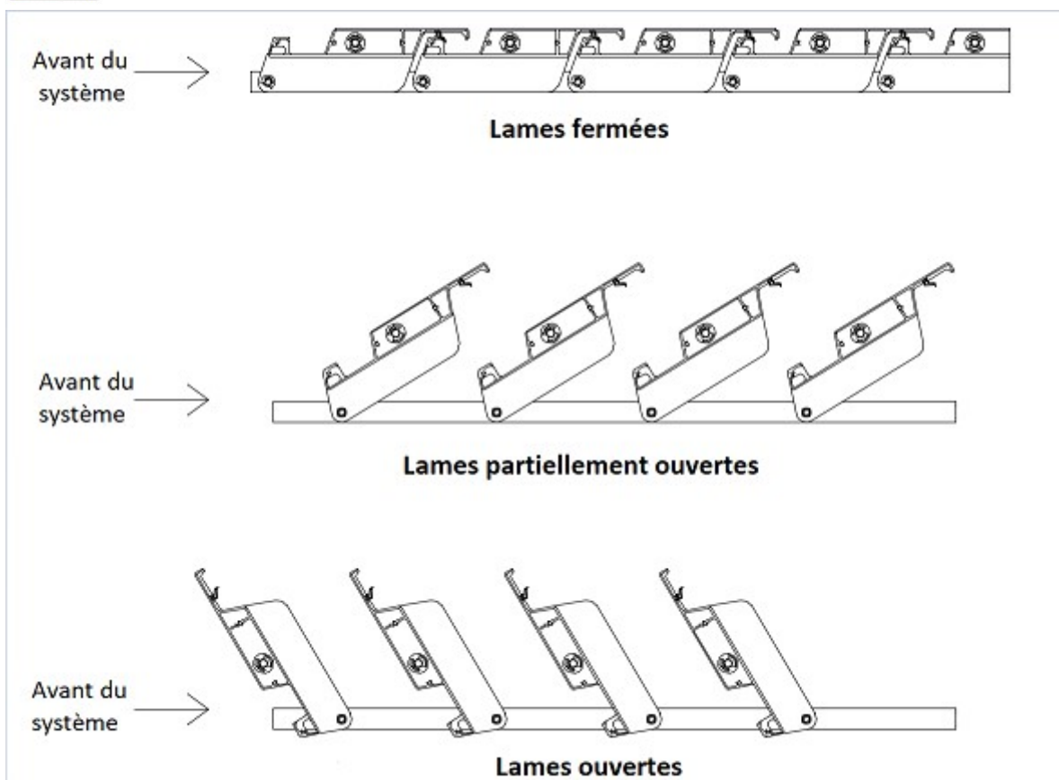
Fig. 2. Réglage standard du sens d'ouverture des lames pour la Pergola SB350 Les dessins sont à titre d'illustration uniquement et ne représentent pas toutes les caractéristiques du produit, entre autres liés à l'utilisation de joints.
