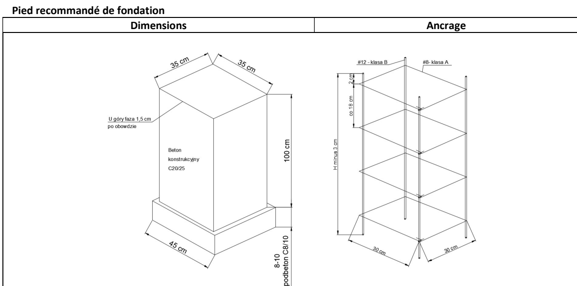
Fig. 34 Forme et renforcement de pied
