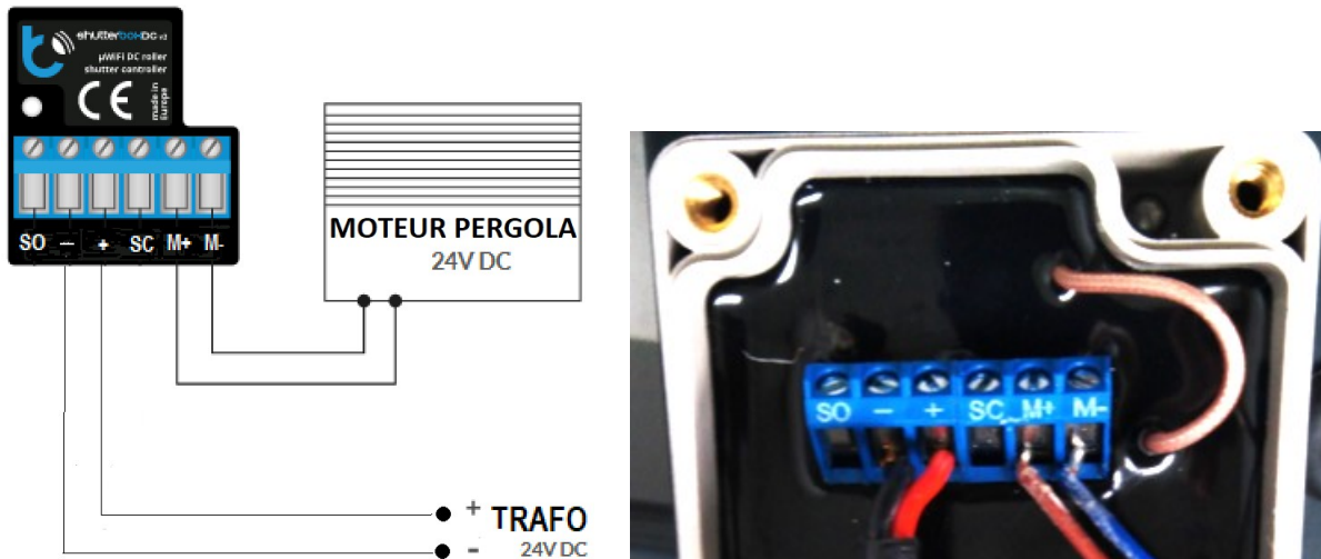
Fig. 36 Schéma de câblage de l'unité de commande Pergola DC (fabriquée par SELT en usine)
